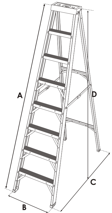
Escalera Abierta
